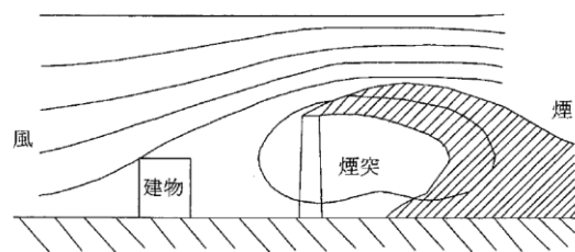
図 7-13 ダウンドラフト現象
