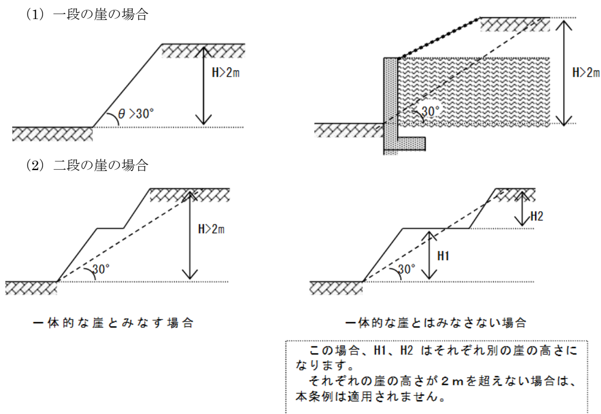
図 9-1 三重県建築基準条例による崖の定義
